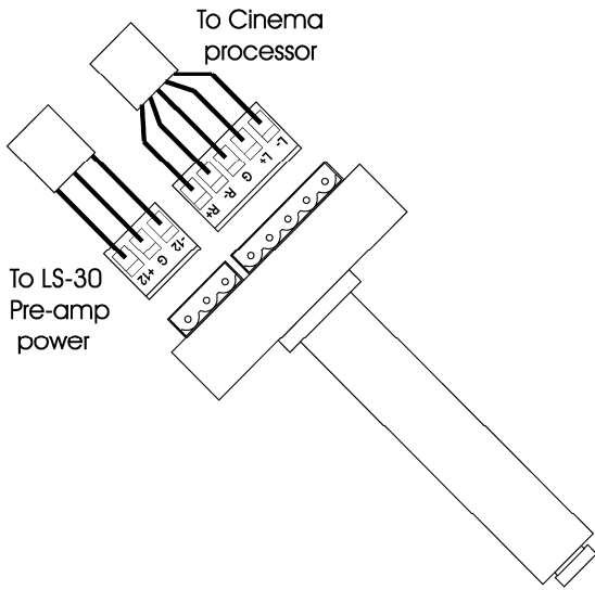
Analog pre-amp
